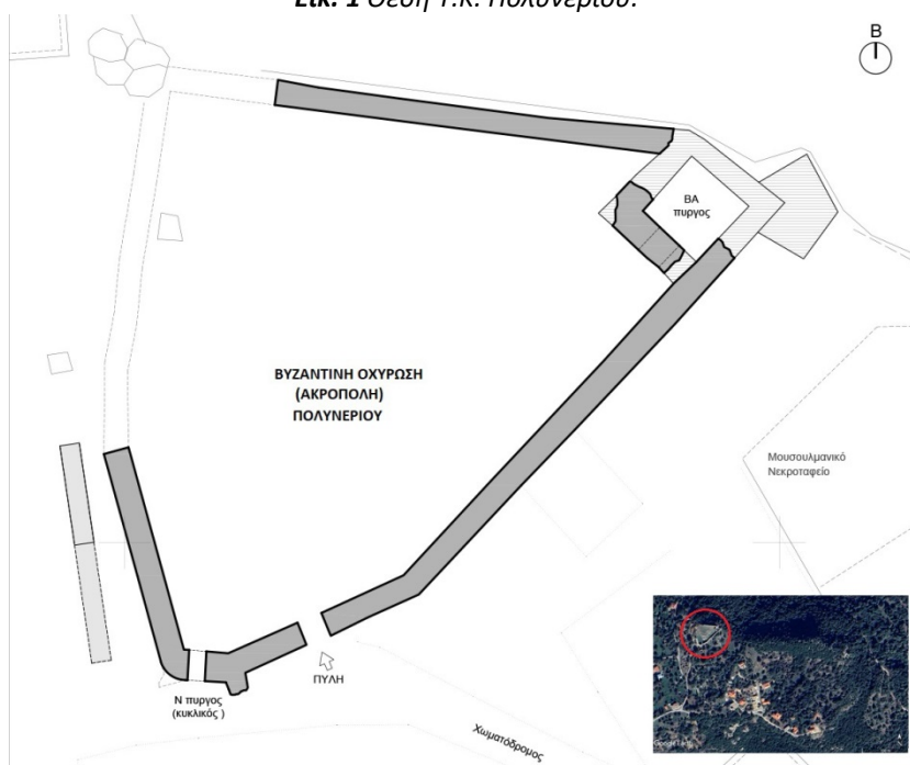
Εικ. 2 Κάτοψη βυζαντινής ακρόπολης κάστρου Πολυνερίου.
